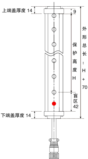
背装L支架尺寸图（mm）
