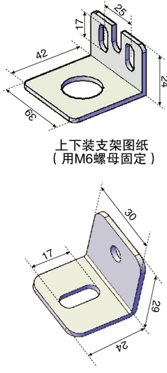
背装支架图纸（用M6螺母固定）
