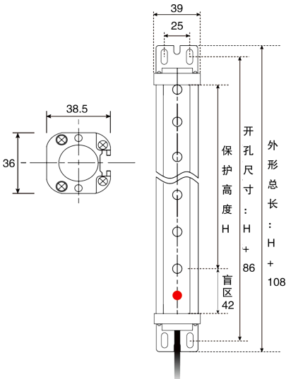
上下正装、侧装L支架尺寸图（mm）
