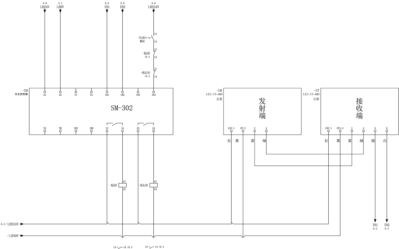
二级光栅接302示意图
