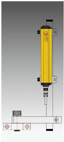
冲压机专用Z型支架-Y
